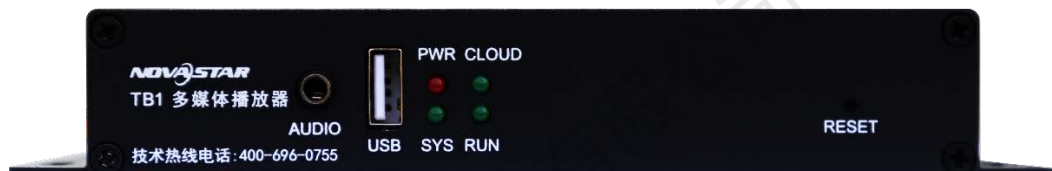
图3-1 TB1 前面板外观
